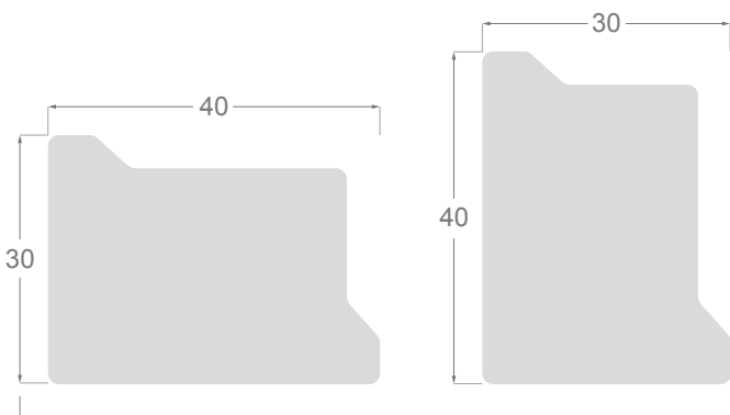
1776/000 Bastidor reversible
