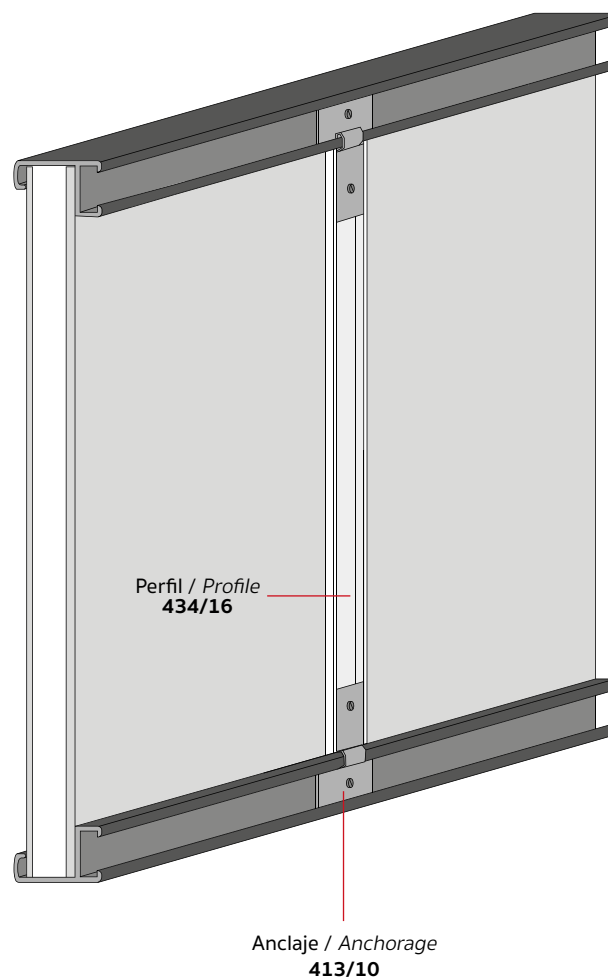
Ejemplo de montaje con perfil estabilizador simple Example of mounting with profile single stabilizer
