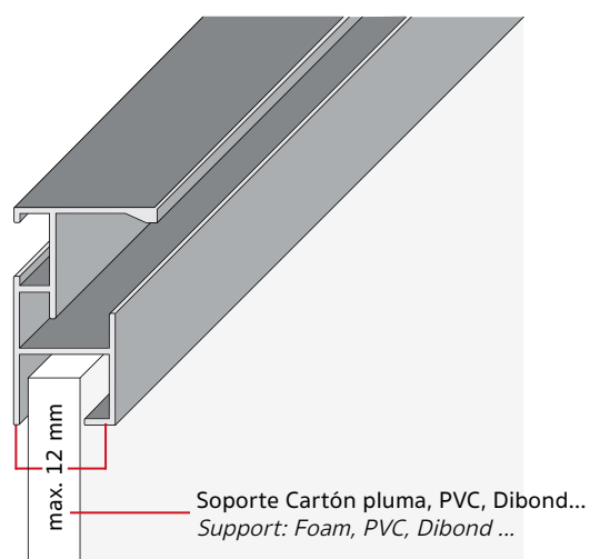
Ejemplo de montaje convencional
