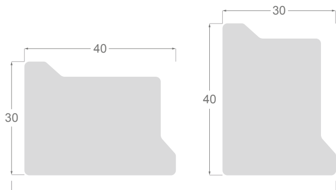
1776/000 Bastidor reversible / Châssis Réversible
