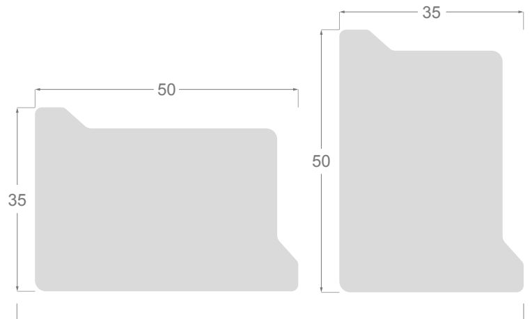
1777/000 Bastidor reversible / Châssis Réversible
