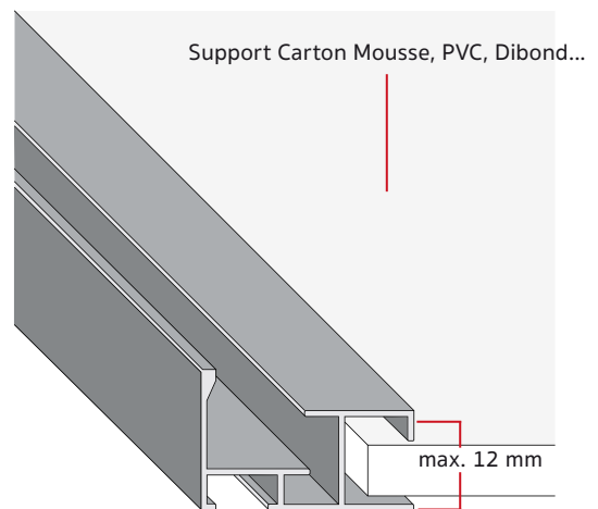
Exemple de montage conventionnel
