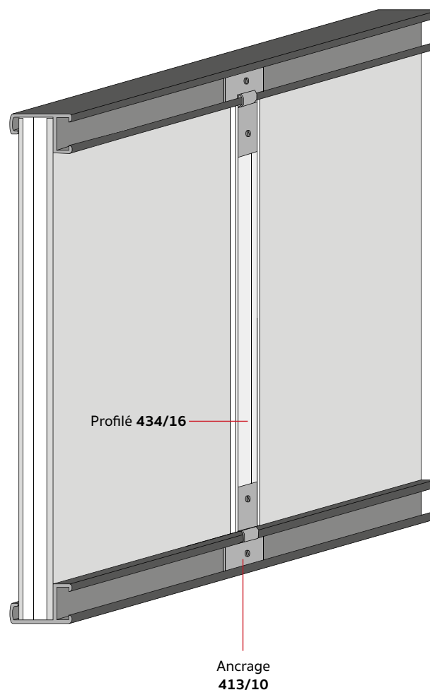
Exemple de montage avec profilé stabilisateur unique
