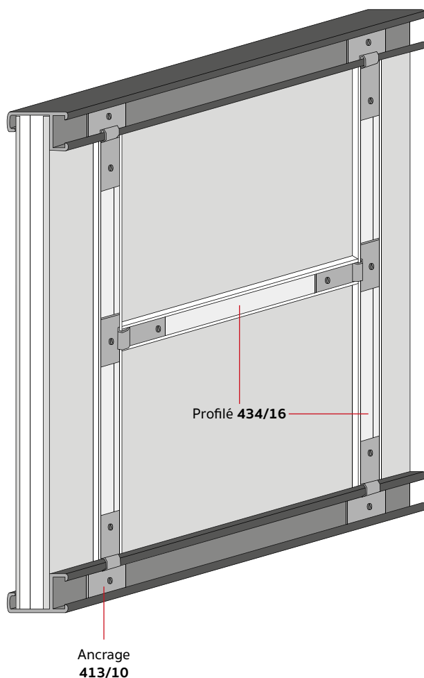
Exemple de montage avec profilé stabilisateur H
