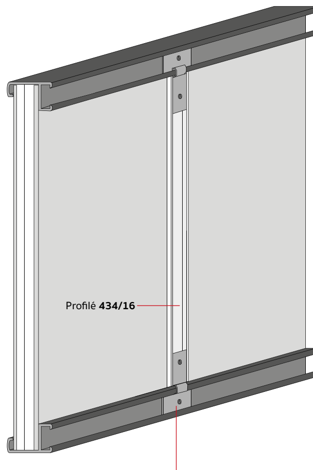
Ancrage 413/10
